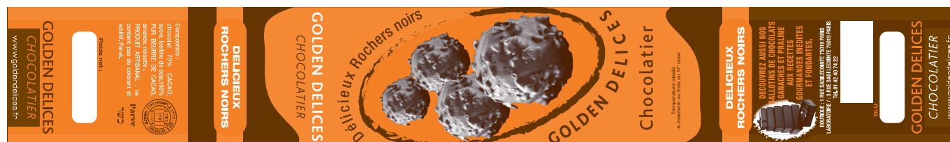
Taille réelle : 290 x 43 mm Réf. E210
